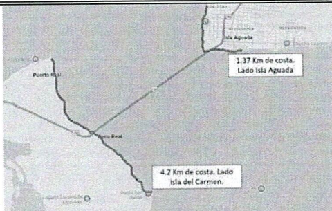
Figura 2: Área de los trabajos de topografía.
